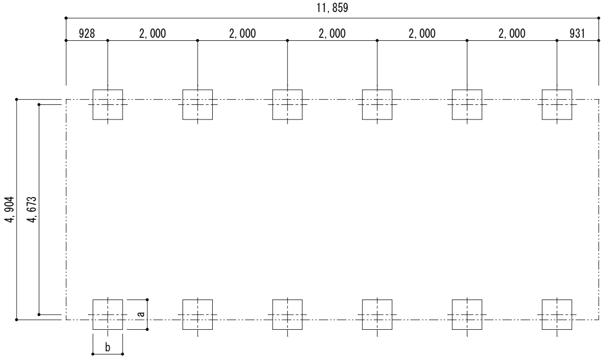
■基礎配置図
